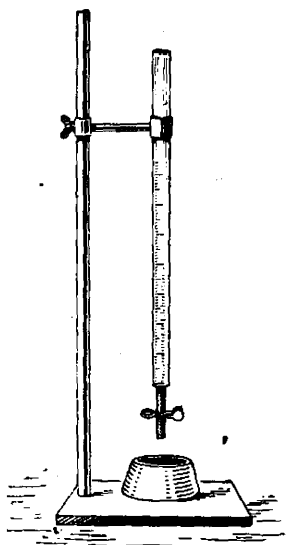
Микробюретка.
